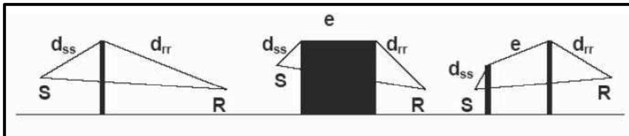
Figura 5 - barriere acustiche
