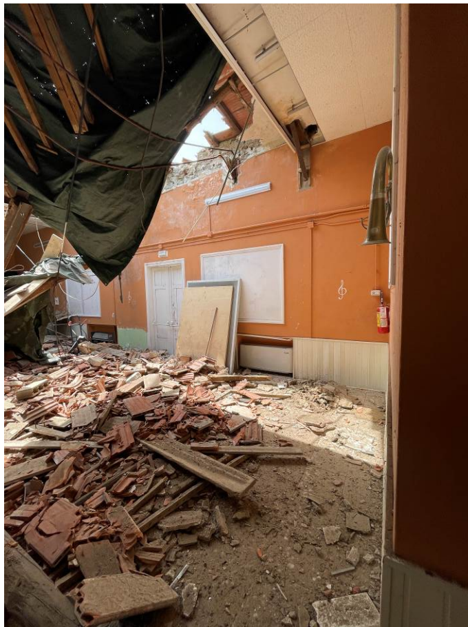
Figura 6 - particolare della capriata C1
