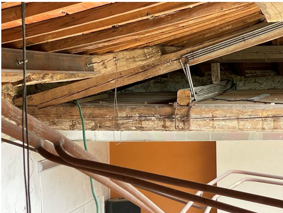
Figura 10 - particolare della capriata C3
