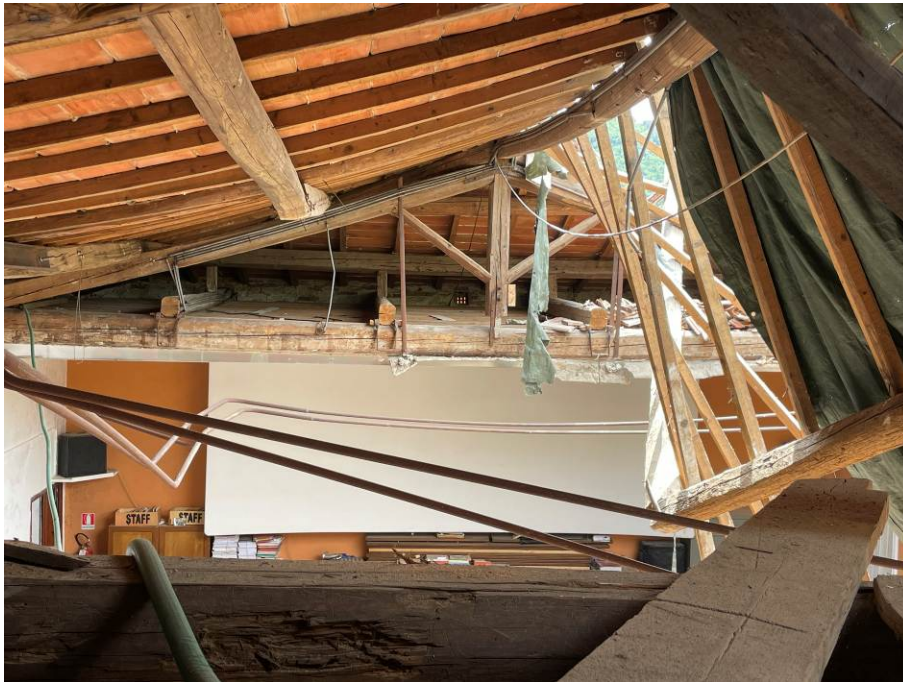
Figura 9 - particolare della capriata C3
