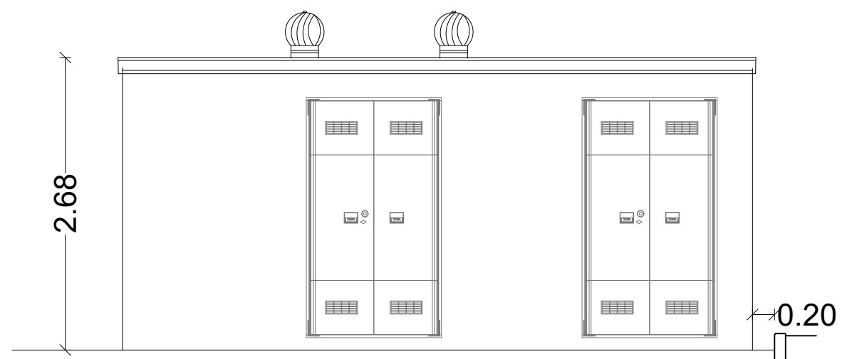
VISTA FRONTALE
