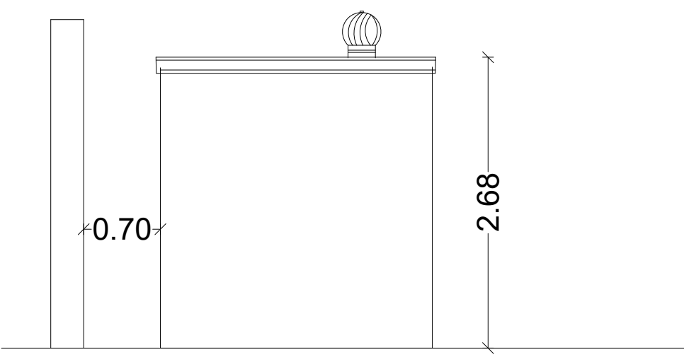
VISTA LATERALE
